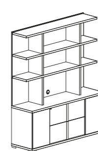
LIBRARY COMPOSITION 10 PJTI0809GR inch W 71" D 20" H 84" cm L 179,6 P 52 H 212,2 Crts 4 kg 242 m 3 1,17
