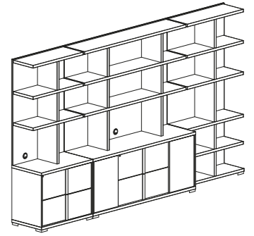
LIBRARY COMPOSITION 4 PJTI0803GR inch W 146" D 20" H 84" cm L 369,4 P 52 H 212,2 Crts 10 kg 468 m 3 2,2
