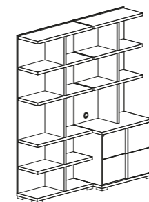
LIBRARY COMPOSITION 13 PJTI0812GR inch W 75" D 20" H 84" cm L 189,8 P 52 H 212,2 Crts 6 kg 226 m 3 1,03
