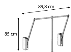
Kit servetto armadi battenti Servetto pull down clothes rack Штанга-вешалка "лифт" д/распашного шкафа
