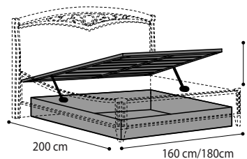
- RETE CONTENITORE CON KIT
