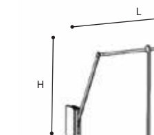
- KIT SERVETTO PER MODULO 2/A ARMADIO BATT. - SERVETTO PULL DOWN CLOTHES RACK FOR 2 DOOR MODULE - ШТАНГА-ВЕШАЛКА "ЛИФТ" Д/РАСПАШНОГО ШКАФА
