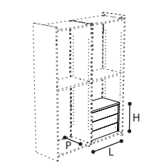
- CASSETTIERA 3 CASSETTI LEGNO PER MOD. 2/A - 3 DRAWERS UNIT FOR 2/D COLUMN - КАССЕТНИЦА 3 ЯЩ.
