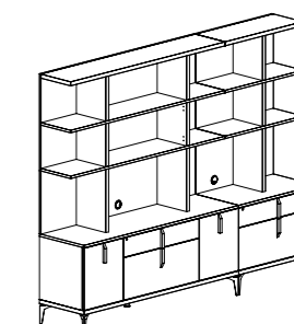
LIBRARY COMPOSITION 8 PJMM0807 inch W 106" D 20" H 84" cm L 270,2 P 52 H 212,2 Crts 7 kg 297 m 3 1,6
